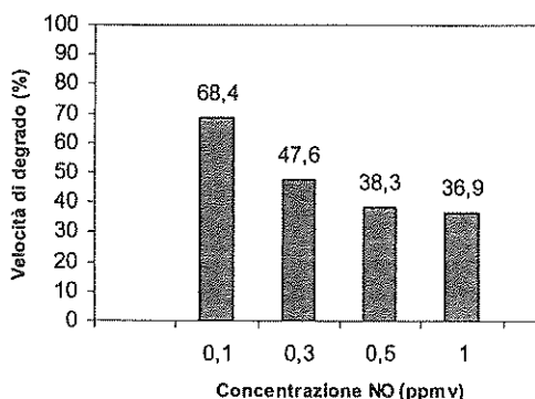
Fig. 2 - Influenza della concentrazione di inquinante sulla velocità di degrado.
