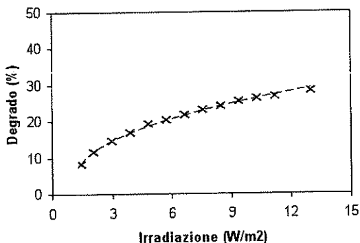
Fig. 3 - Influenza dell'irradiazione sulla velocità di degrado.
