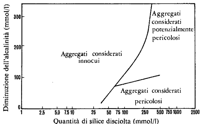
Fig.1 - Valutazione della reattività dell'aggregato. Diminuzione dell'alcalinità in funzione della silice disciolta.
