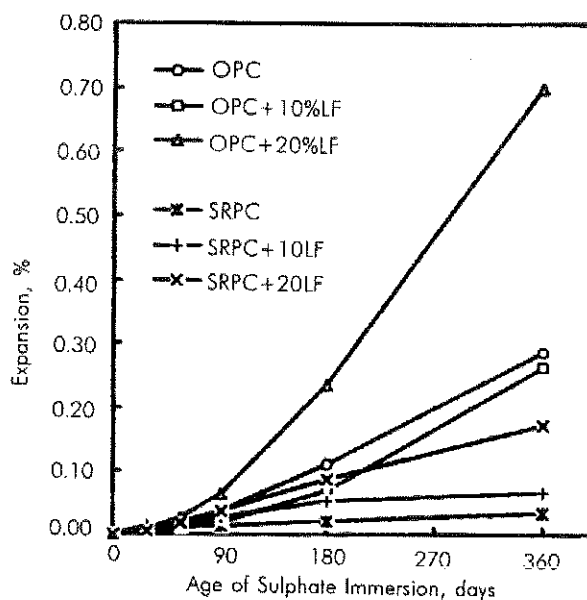
Fig. 1 – Espansione di cemento Portland ordinario e di cemento Portland resistente ai solfati, contenente 10% o 20% di filler calcareo, esposti fino a 360 giorni ad una soluzione di solfato sodico (7)
