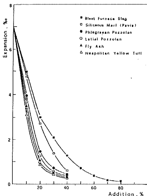
Fig. 2 - Espansione di barre di malta in funzione del tipo e del tenore di prodotto cementizio supplementare, al termine di due anni (6).
