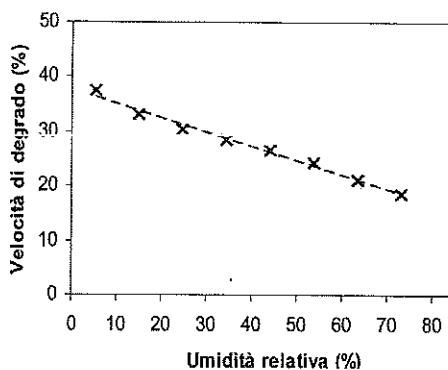
Fig. 1 - Influenza dell'umidità relativa sulla velocità di degrado.
